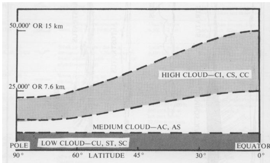
Figure 30 - Cloud Heights and Latitude
